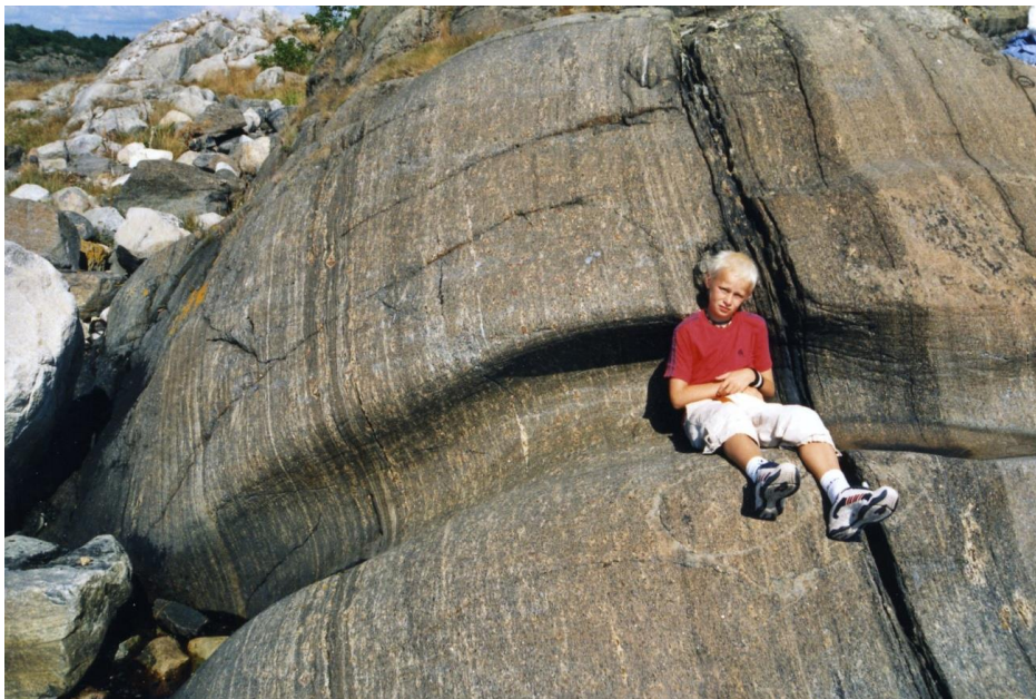
Figur 37. Renneformer på øyene utenfor Hasseltangen. Isskuring inne i formene er synlig. Foto: IJJ
