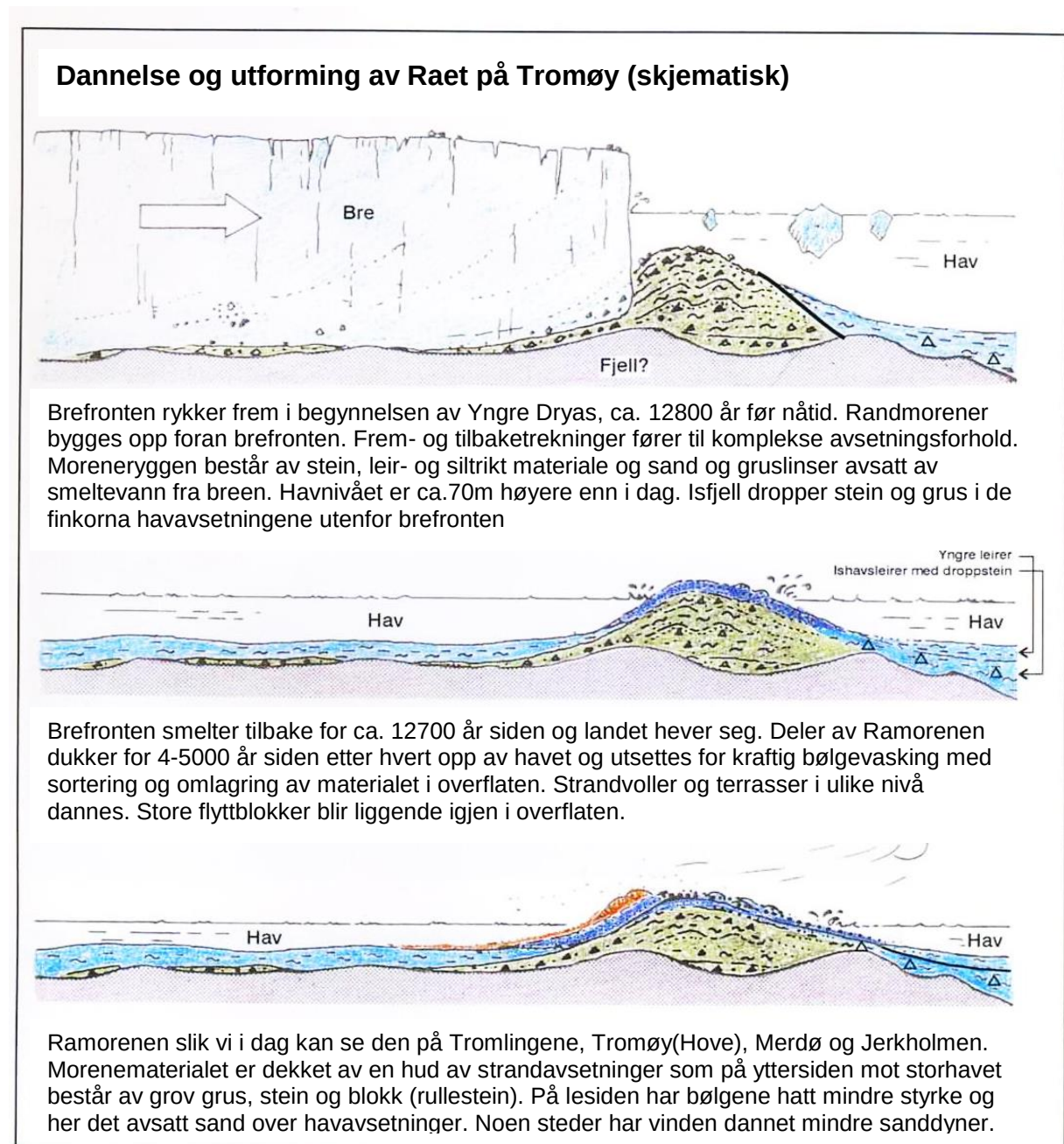
Figur 63. Dannelsen av Raet på Tromøy. Fig: IJJ
