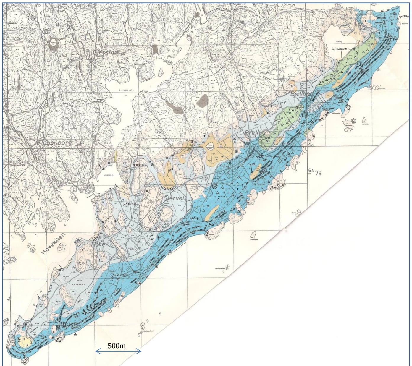
Figur 77. Raet-Botne-Hove. Kvartærgeologisk oversiktskart: For tegnforklaring, se vedlegg 1.
