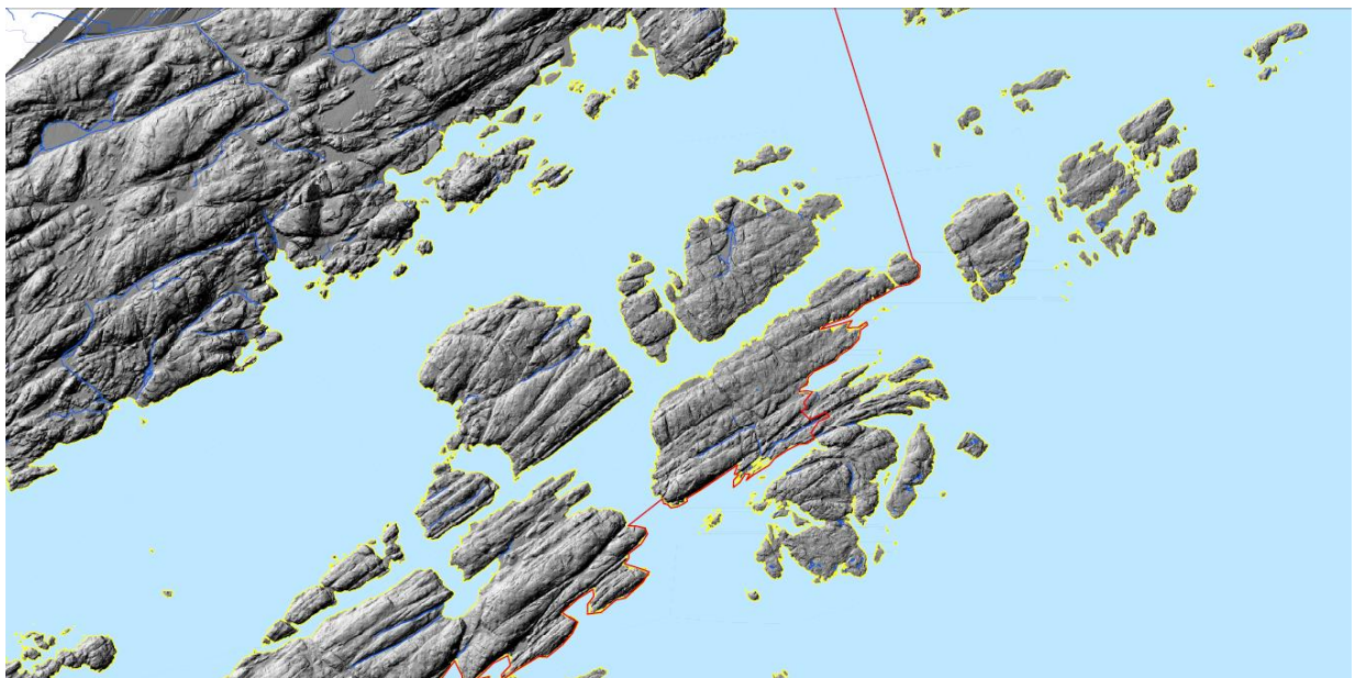
Figur 16. Furet og værbit! Laserdata med terrengskygge viser berggrunnstrukturene, strøkretning og sprekker tydelig. Kilde: Geovekst/Aust-Agder fylkeskommune
