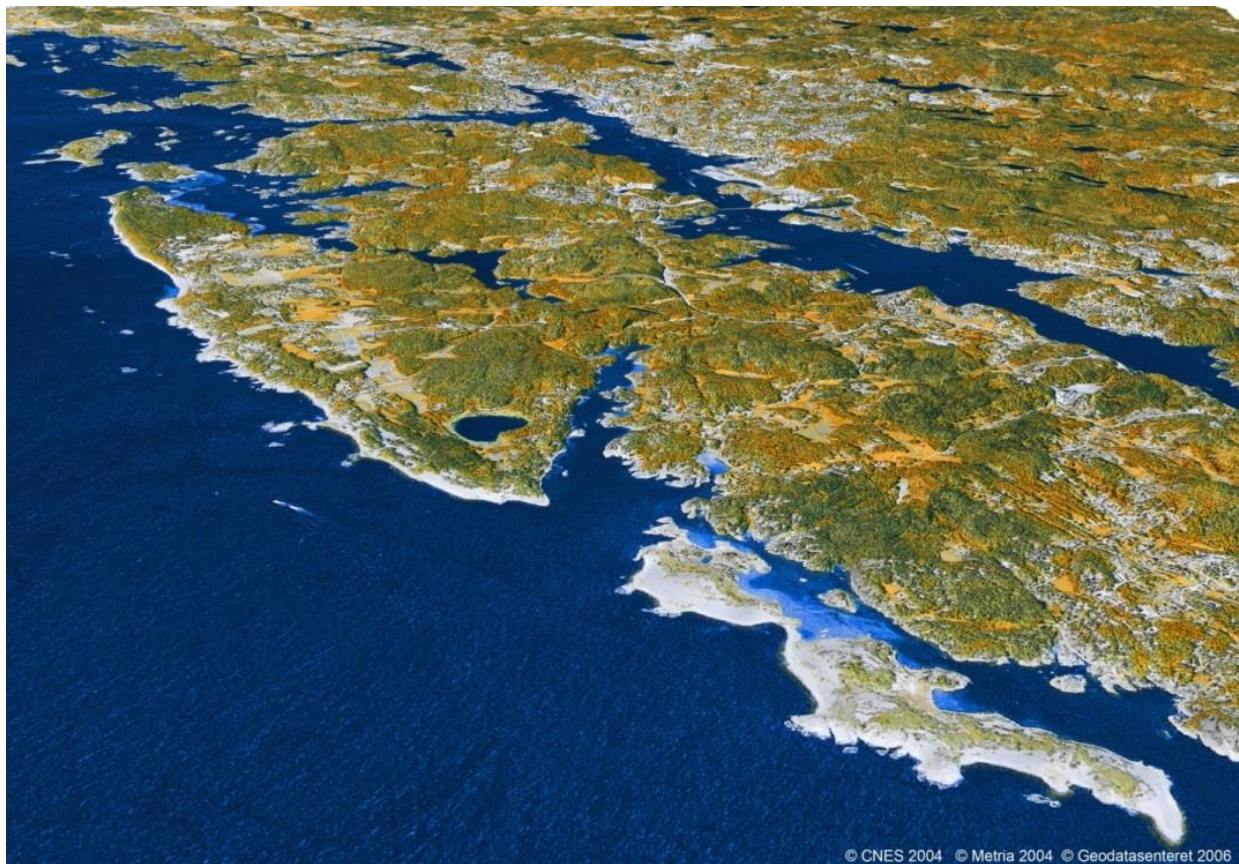
Figur 64. Satellittbilde i 3D. Tromøy- «øya med bremmen». Fra Tromlingene, Botne – Hove. Arendal by i bakgrunnen. Kilde: Geodatasenteret/Asplan Viak.
