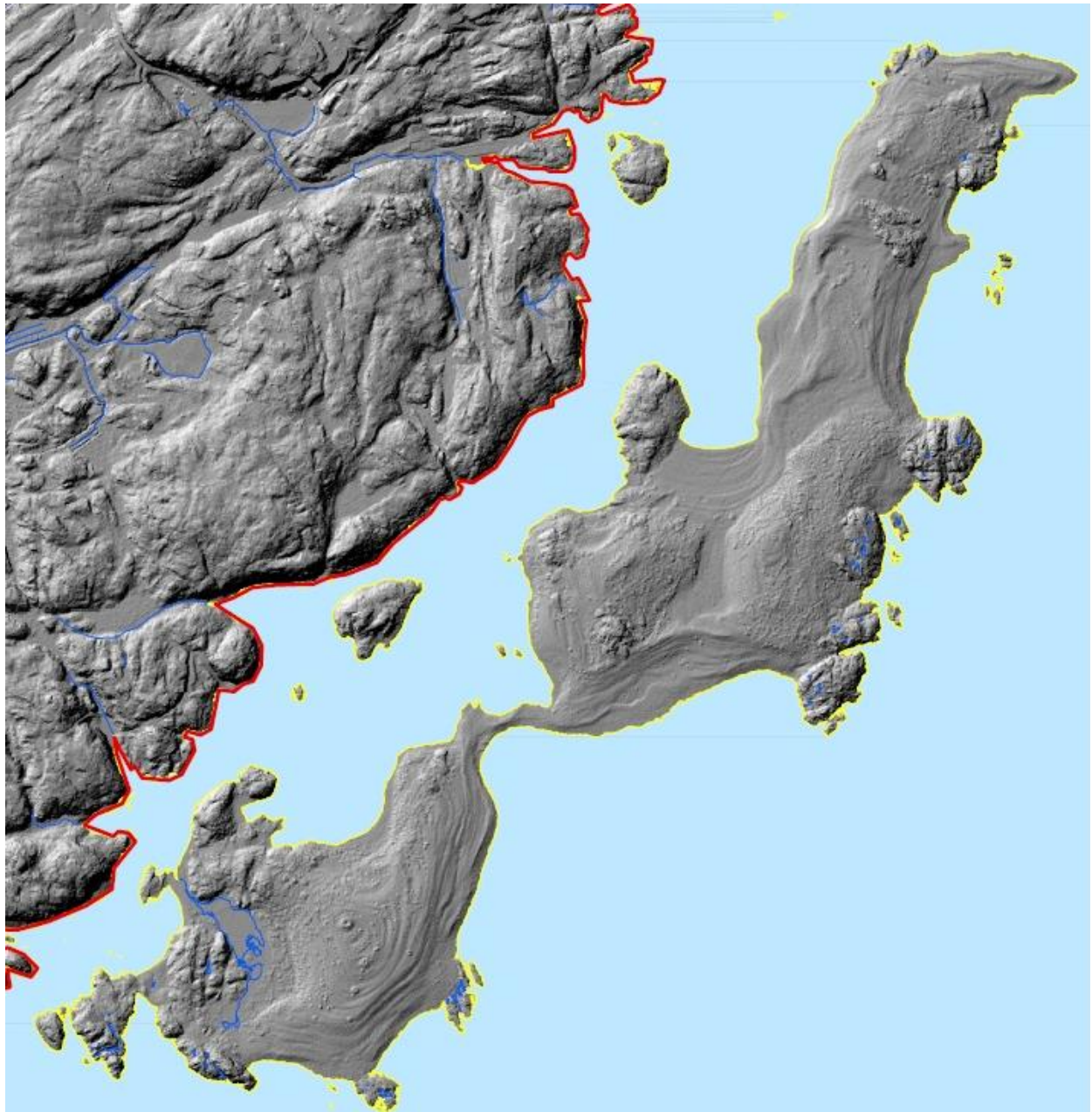
Figur 57. Tromlingene. Utsnitt av laserkart-terrenkskygge. Strandvollene vises særlig tydelig, men ikke alltid der det er tett krattvegetasjon. Også områder med mer inntakt Ramorene som ligger i le bak oppstikkende fjell synes godt. Flere gravrøyser er synlige.
