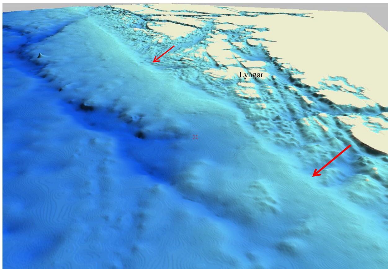
Figur 26. 3D modell av sjøbunnsdata. Ramorenen i sjøen utenfor Lyngør. Legg merke til at innsiden av Raet i stor grad er renskrappt for løsmasser som nå ligger i Ramorenen. Utenfor Raet er sjøbunnen utjevnet av sedimenter. Iskontaktsiden, mot land, av Raet er tydelig brattere enn utsiden. Piler vis isbevegelsesretning. Kilde: Geodatasenteret/Asplan Viak
