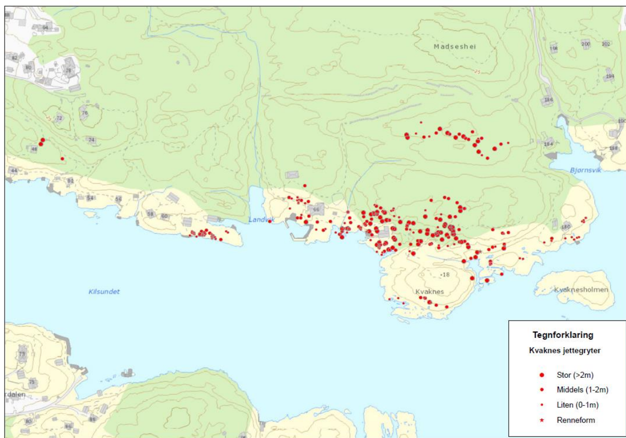
Figur 51. Kartoversikt over Kvaknesområdet
