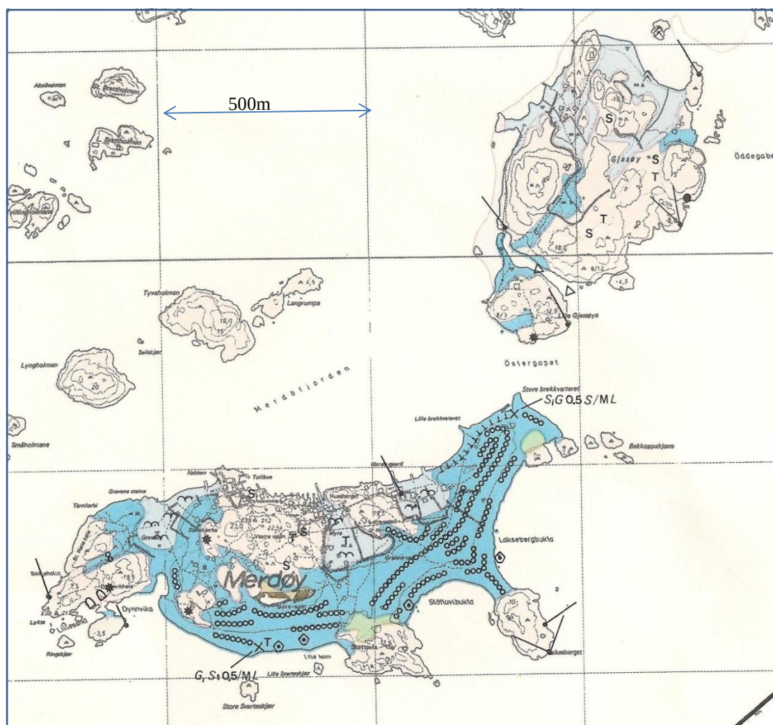
Figur 78. Merdø. Kvartærgeologisk oversikt. For tegnforklaring, se vedlegg 1.
