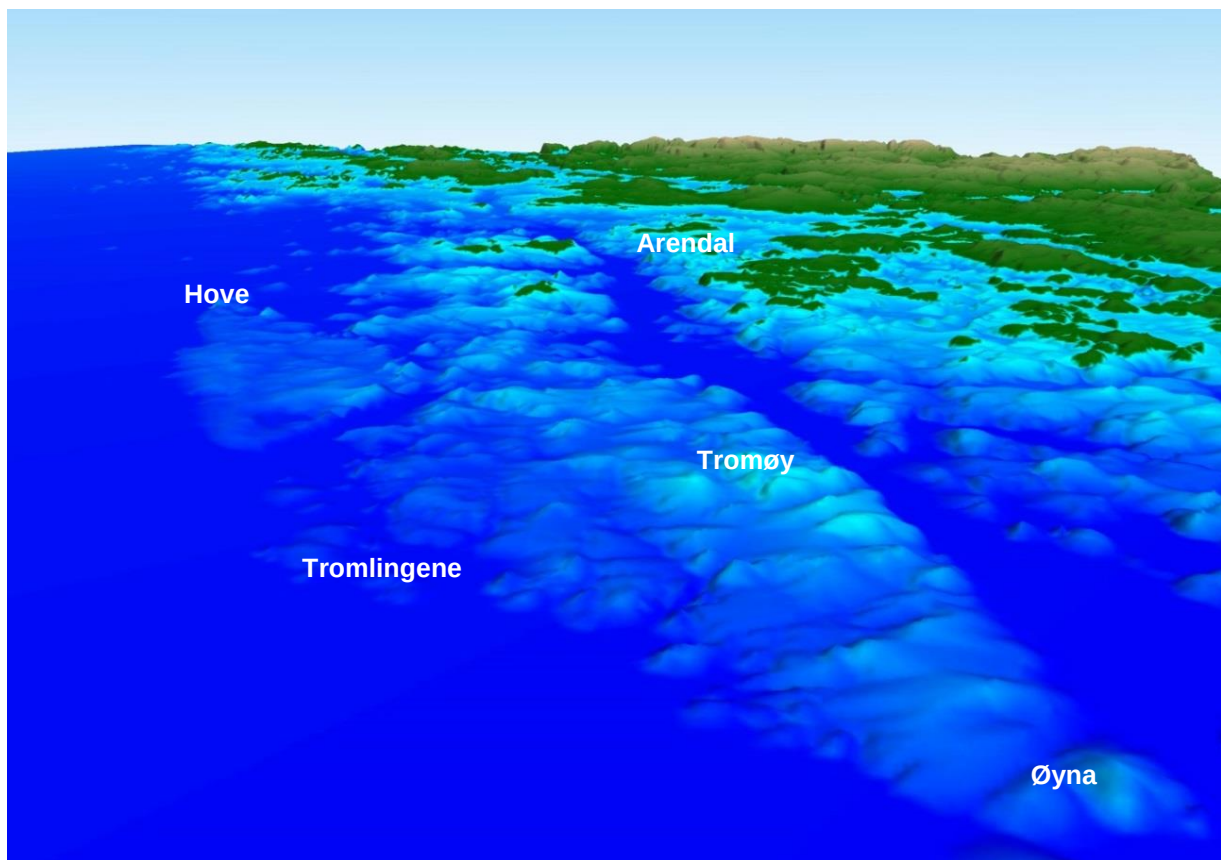
Figur 40. Havets høyeste nivå. Oversiktsbilde av Tromsø sett fra nordøst. Havnivå ca. 70 m høyere enn i dag. Kilde: Geodatasenteret/Asplan Viak
