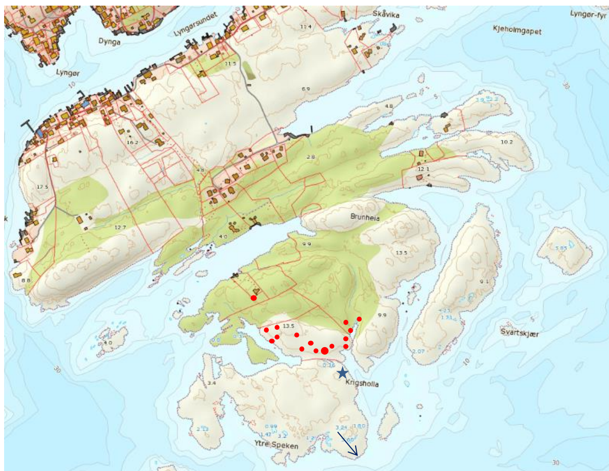
Figur 49. Kartutsnitt Krigsholla, Ytre Lyngør. Jettegryter markert med rødt. Krigsholla er den største. Blå stjerne er område med renneformer, som det også er flere andre steder. Pil markerer isskuringsretning.
