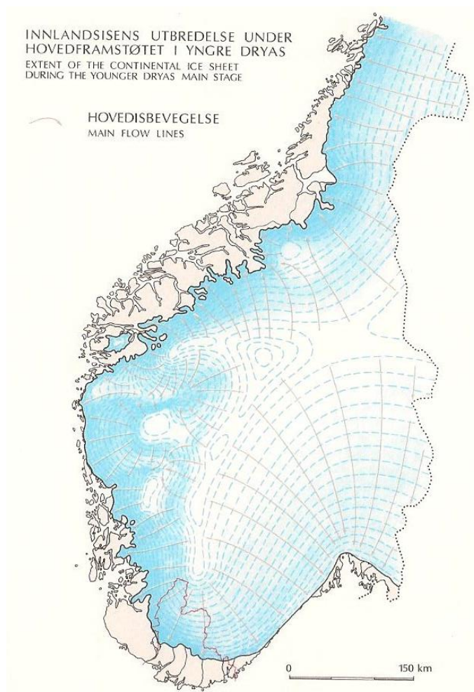
Figur 25. Isdekke og isbevegelse i Yngre Dryas. Kilde: Sollid, J.L. & Sørbel, L. 1981
