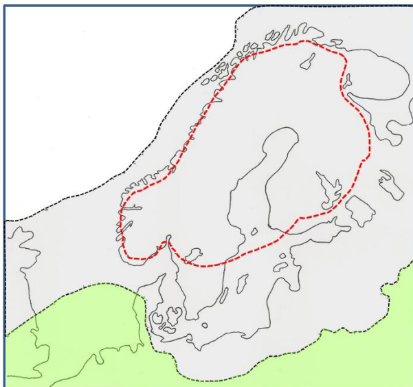
Figur 19. Skandinavia under siste istid.
