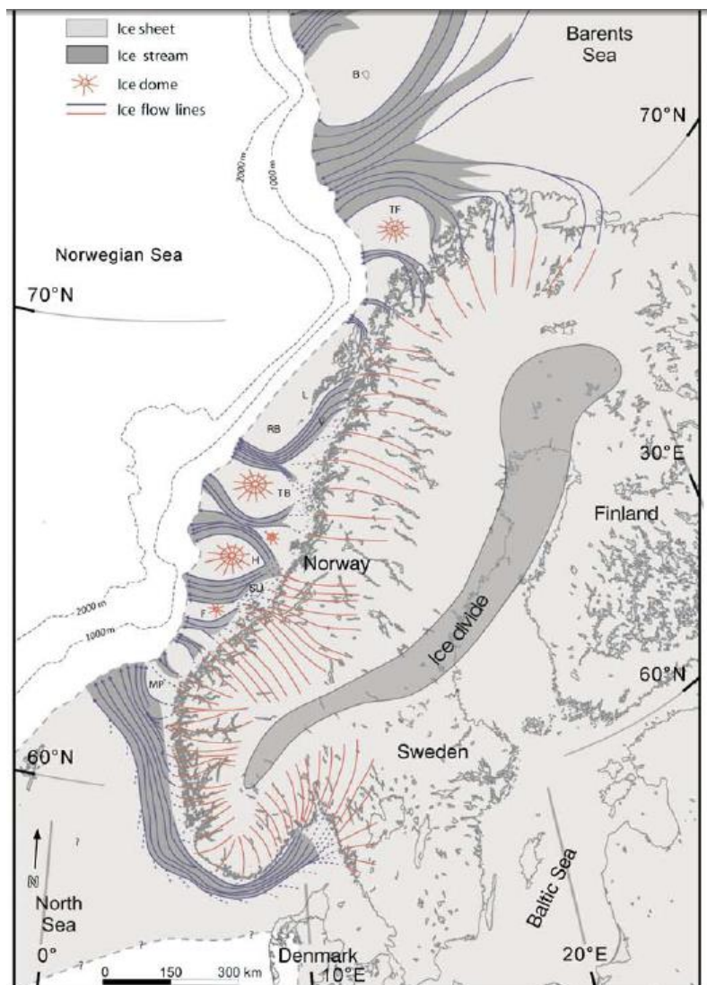
Figur 23. Oversikt over isbevegelse/isstrømmer over Skandinavia når isdekket hadde sin største utbredelse. Merk den markerte isstrømmen ut gjennom Skagerrak. Kilde: D. Ottesen m.fl. NGU
