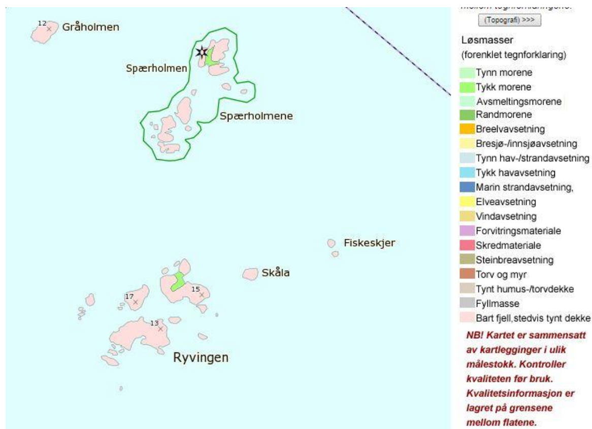
Figur 106. Spærholmene (til venstre) og Ryvingen. Kilde: Utsnitt fra NGU's database
