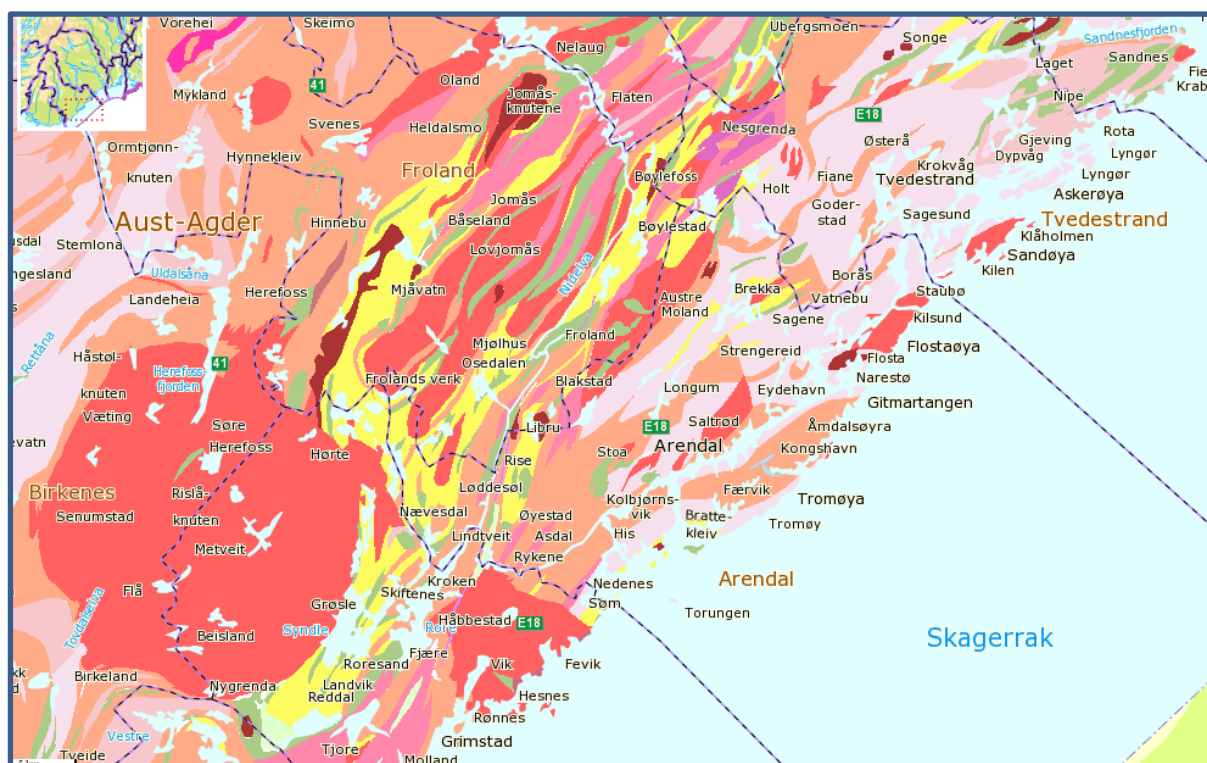
Figur 3. Berggrunnsgeologisk oversikt - utsnitt fra NGU's database. Rødt er granitt, gult er kvartsitt, grønt er gabbro og amfibolitt, lysebrunt og lilla er ulike gneiser. Kartutsnittet ovenfor er en oversikt basert på kart i M1:250 000. Detaljerte kart fra kartlegging i M 1:50 000 finnes for kystområdene i Aust-Agder (Vedlegg 3). For nærmere info om de ulike bergartene se NGU's kartjeneste; www.ngu.no
