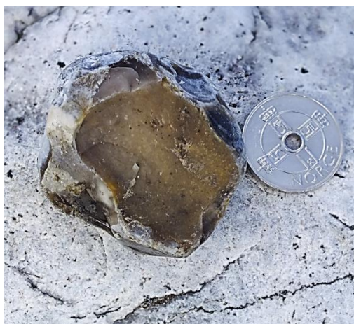
Figur 76. Rullesteinsområdene inneholder en fantastisk samling bergarter fra store deler av Sør-øst Norge, her er rombeporfyr, kalkstein fra kambro-silur, flint (fra Danmark?) og larvikitt fra Vestfold. Foto: IJJ
