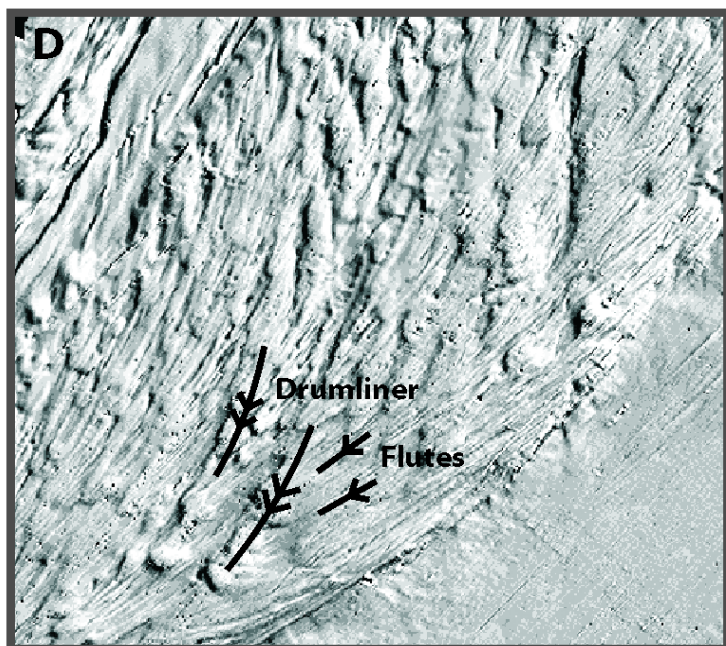
Figur 24. Flutings og drumliners på bunnen av Skagerrak, ca. 20km sørøst for Arendal viser tydelige spor fra en stor isstrøm fra nordøst, - ut gjennom norskerenna. Data fra multistråleekkolodd.
