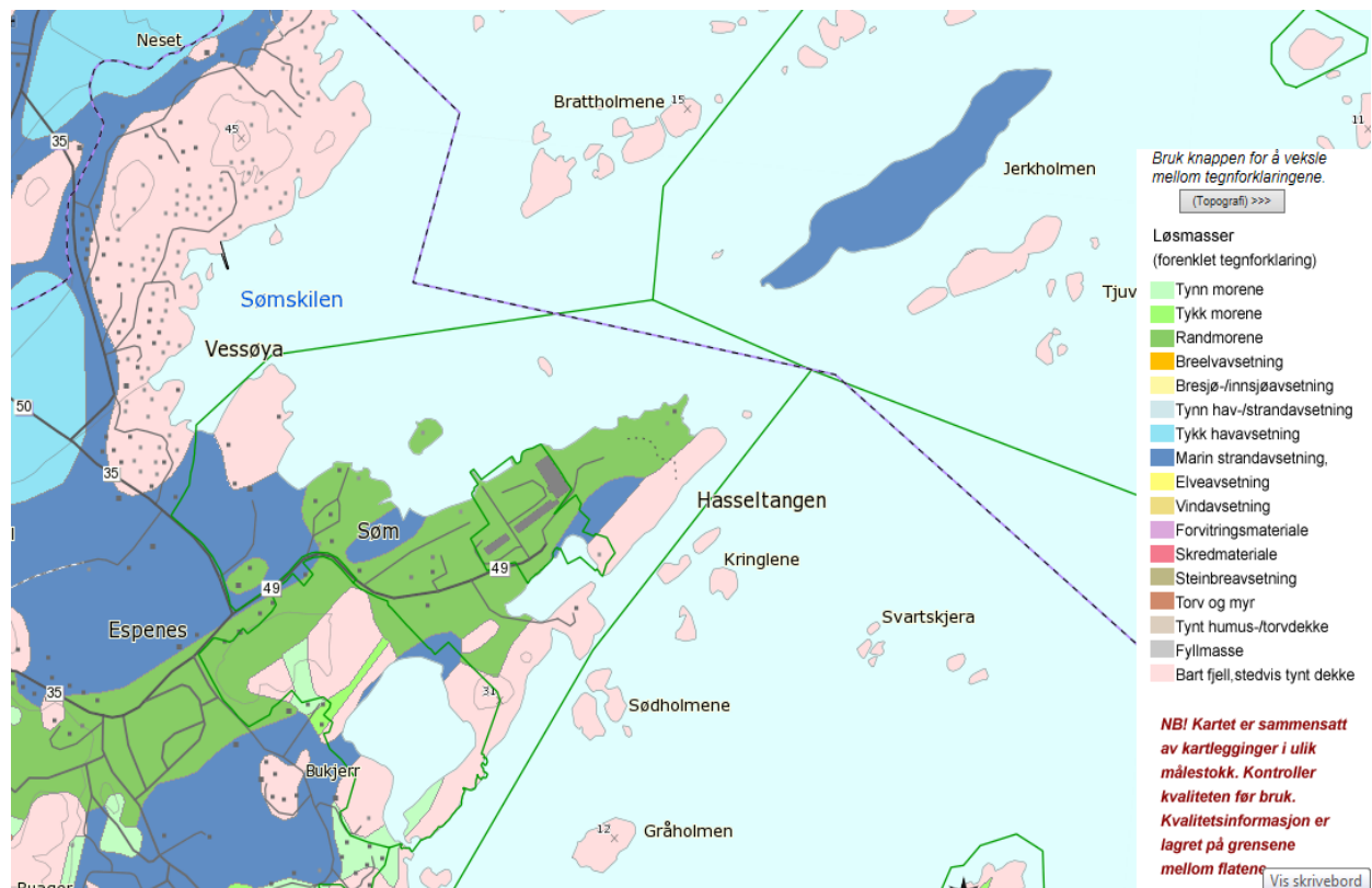
Figur 92. Kvartærgeologisk oversiktskart: Kilde: NGU's kartdatabase/ løsmasser.
