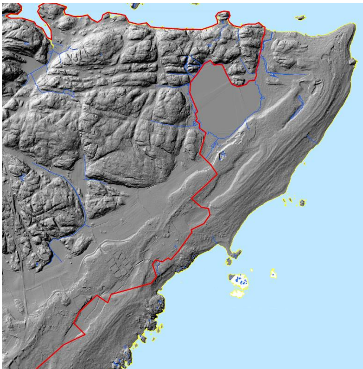
Figur 66. Botne-Bjellandstrand. Laserkart-terrengskygge viser form og strandvoller på Raet. Her sees 2 parallelle morenerygger, den ytterste er mest bearbeidet av bølgene, med strandvoller. Inngrep, tidl. grustak, sees bl.a. ute ved nordøstpynten ved Botne. Kilde: Geovekst/Aust-Agder fylkeskommune
