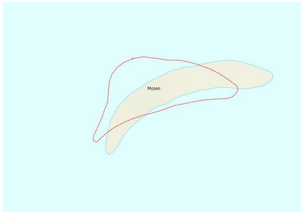
Figur 27. Molen utenfor Flosta. Raet dukker opp av sjøen som en steingrunne ca. 2 km fra land, men endres stadig av bølgenes arbeid. Grå farge viser omriset i 2009 mens rødt omriss viser formen på øya i 2012.
