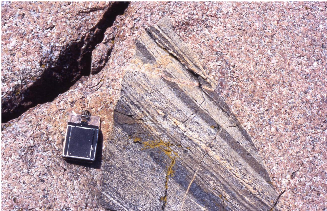
Figur 110. Bruddstykker av gneis innesmeltet i granitt forteller om en dramatisk hendelse, dypt i jordskorpa for over 900 mill. år siden. Foto: IJJ.
