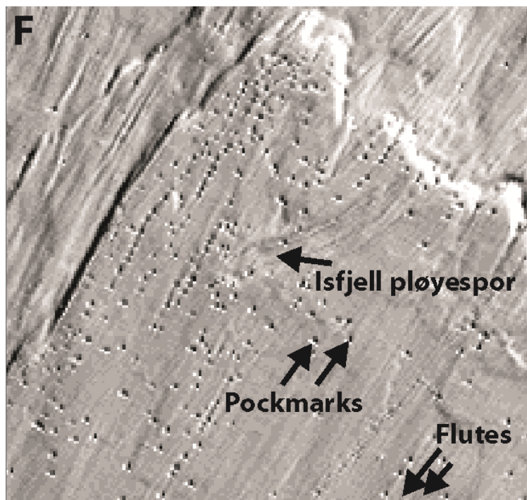
Figur 12. Såkalte pockmarks fra Skagerrak, små kratere som indikerer utslipp av grunn gass eller væske. Multistråle-ekkolodd-data. Kilde: Landet blir til- 2006. Modifisert etter O. Longva og T. Thorsnes, NGU
