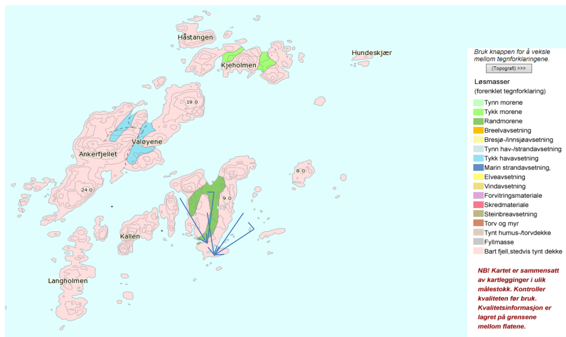
Figur 107. Kartutsnitt – Valøylene. Fra NGU's kartdatabase. I tillegg er iskurings-retninger lagt inn (blå piler)
