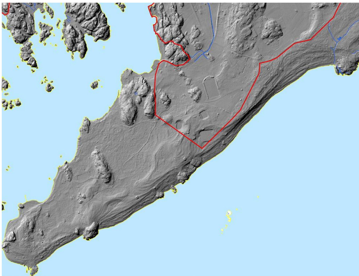
Figur 67. Spornes-Hoveodden. Laser-terrengskygge kart. Strandvollssystemene er godt synlige, men kan være kamuflert i tett skog/kratt. Oppstikkende fjell og flere gravhauger sees tydelig. Kilde: Geovekst/Aust-Agder fylkeskommune
