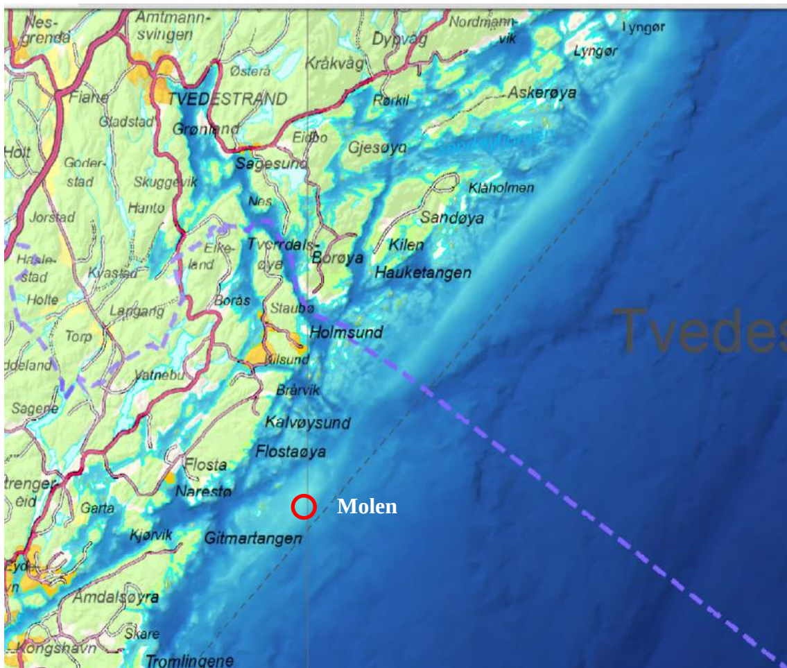
Figur 28. Oversiktskart som viser Raet som en lys linje i sjøen utenfor Aust - Agder . Kilde: norgeskart.no
