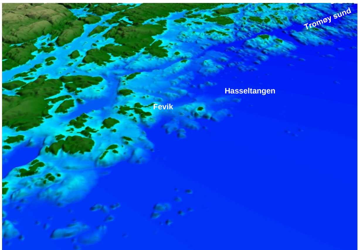
Figur 41. Havnivå etter at isen smeltet bort fra området. 3Dkart fra Fevik-Hasseltangen-med Arendal-Hisøy i bakgrunnen. Havnivå på Hasseltangen ca. 60 moh. Kilde: Geodatasenteret/Asplan Viak
