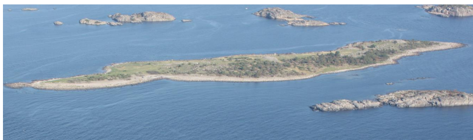
Figur 88. Oversiktsfoto av Jerkholmen. Kilde: Geovekst/Kartverket
