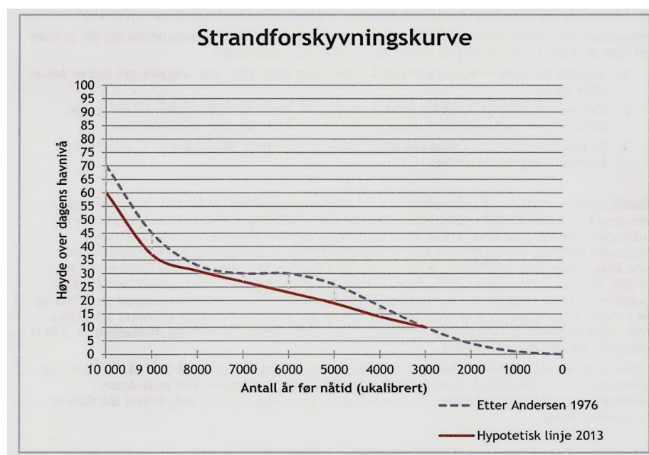
Figur 42. Strandforskyvningskurver. Kilde: Eskeland, K. m.fl. 2012-2013. Rapport fra kulturhistorisk registrering.
